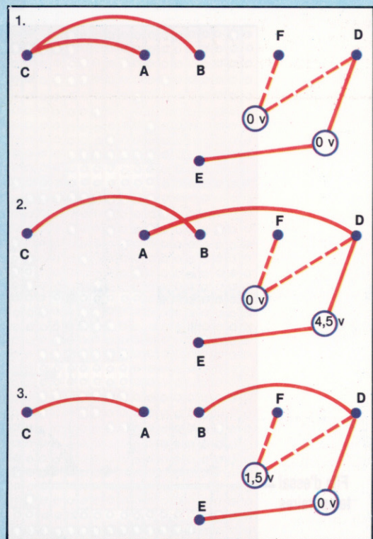
Ce diagramme montre les connexions d'essai qui doivent être établies entre les points A, B, C et D, et les lectures obtenues aux points E et F lors de chacune des trois étapes d'essai.
